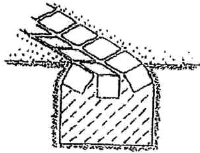
Zuleitung als Natursteinrinne
