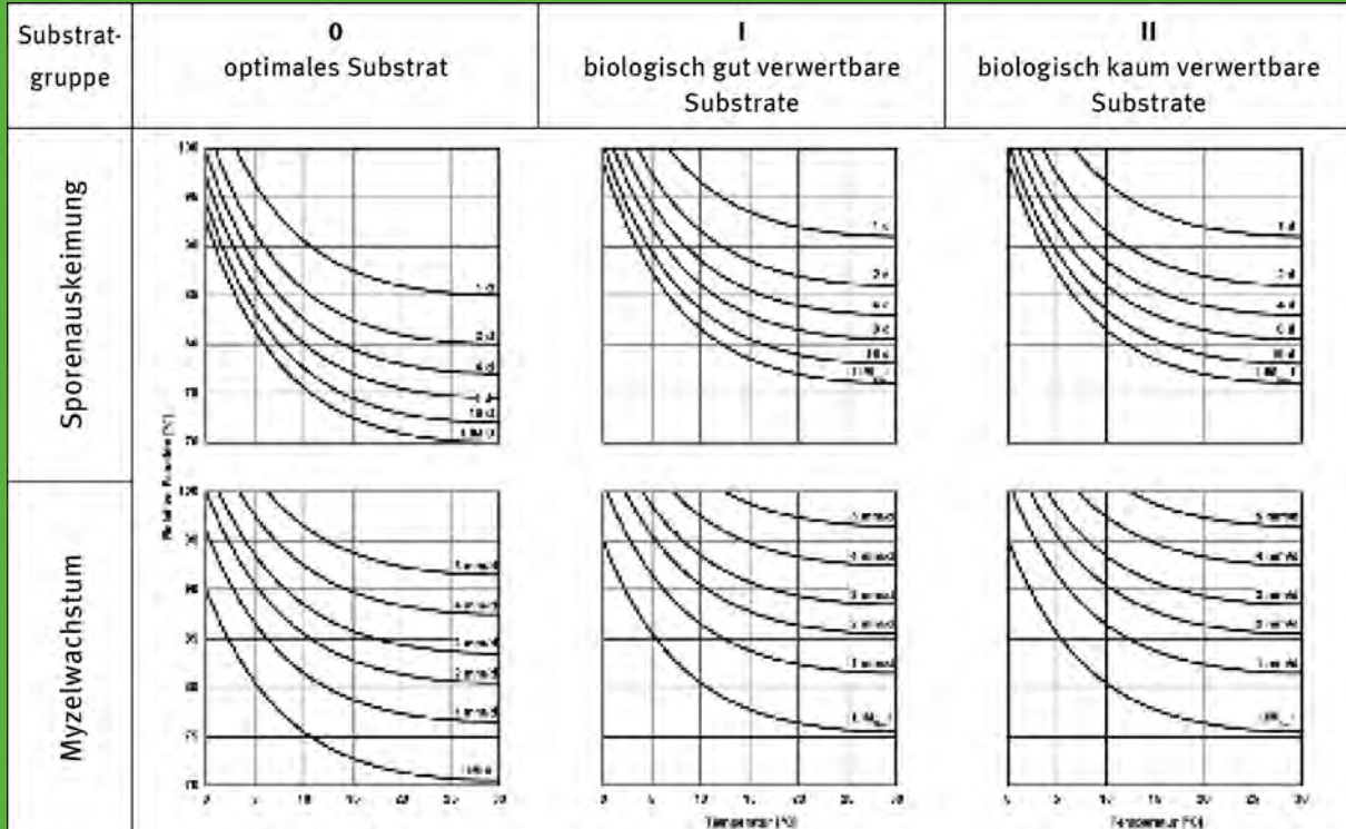
Verallgemeinerte Isoplethensysteme für die Sporenauskeimung (oben) und Myzelwachstum (unten), die für in Bauteilen auftretenden Pilze gelten (nach Sedlbauer 2001); für optimales Substrat (links), für Substratgruppe I (mittig) und für Substratgruppe II (rechts). Die angegebenen Werte charakterisieren die Zeitdauer in Tagen, nach welcher eine Keimung abgeschlossen ist, bzw. das zu erwartende Wachstum in mm/Tag. LIM (Lowest Isopleth for Mould) zeigt die unterste Grenze der Sporenauskeimung bzw. des Myzelwachstums an.
